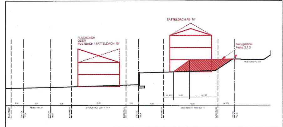
Abb.: Geländeschnitt (Systemschnitt) (Bensing + Partner, 01/ 2025), ohne Maßstab
